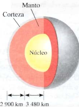
Estructura interna de la Tierra
