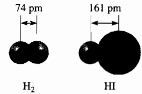
FIGURA 9.3 Longitudes de enlace de las moléculas de \text{H}_2 y \text{HI} .
