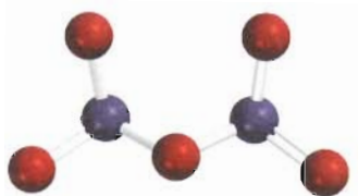
\text{N}_2\text{O}_5
