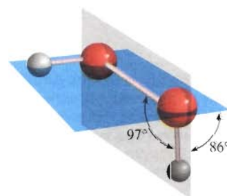
FIGURA 21.12 Estructura del \text{H}_2\text{O}_2 .
