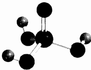
H 3 PO 4
