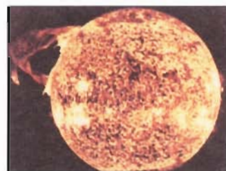
FIGURA 23.14 La fusión nuclear mantiene la temperatura interior del Sol a unos 15 millones de °C.
