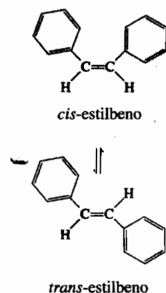
FIGURA 14.5 Equilibrio entre cis -estilbeno y trans -estilbeno. Observe que ambas moléculas tienen la misma fórmula molecular ( \text{C}_{14}\text{H}_{12} ) y también el mismo tipo de enlaces. Sin embargo, en el cis -estilbeno, los anillos de benceno se encuentran en un lado del enlace \text{C}=\text{C} y los átomos de H en el otro lado, mientras que en el trans -estilbeno, los anillos de benceno y los átomos de H se encuentran en lados opuestos del enlace \text{C}=\text{C} . Estos compuestos tienen diferentes puntos de ebullición y momentos dipolares.
