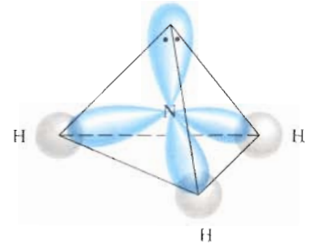
FIGURA 10.9 El átomo de N con hibridación sp^3 en el \text{NH}_3 . Tres orbitales híbridos sp^3 forman enlaces con los átomos de H. El cuarto orbital está ocupado por el par libre del nitrógeno.
